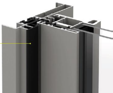
Cache thermique d'isolation et de finition
