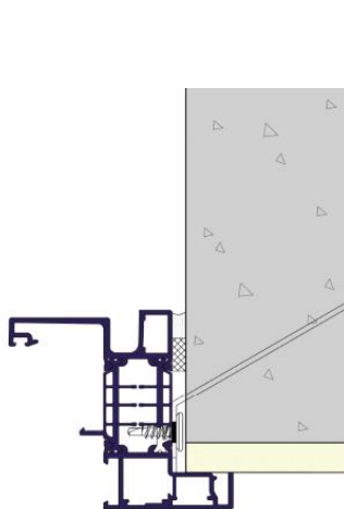
POSE EN TUNNEL AFFLEURANT SANS CORNIÈRE
