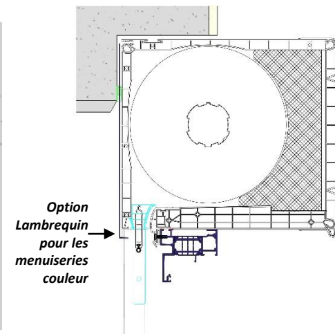
BLOC-BAIE EN FEUILLURE
