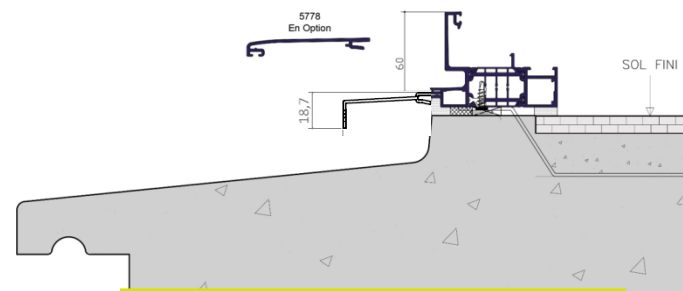
Seuil SANS RECOUVREMENT
