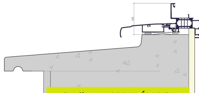
Seuil avec APPUI ÉLARGI
